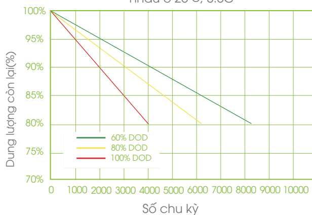
Đường cong tuổi thọ ở các độ sâu xả khác nhau ở 25°C, 0.5C
