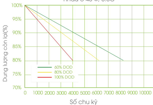
Đường cong tuổi thọ ở các độ sâu xả khác nhau ở 40°C, 0.5C
